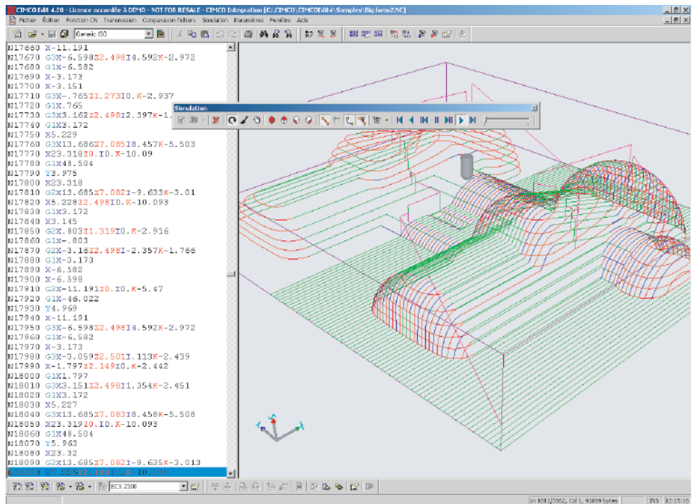
Cimco Edit et la simulation (en option) du programme CN
